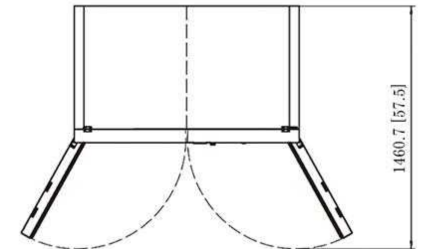
Door open size
